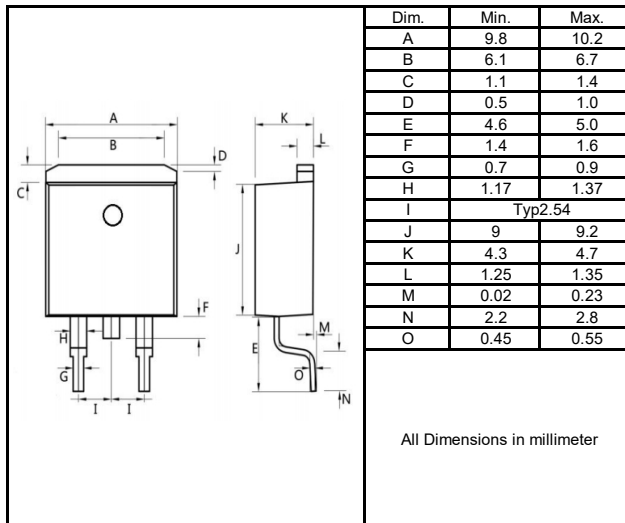
TO-263C
